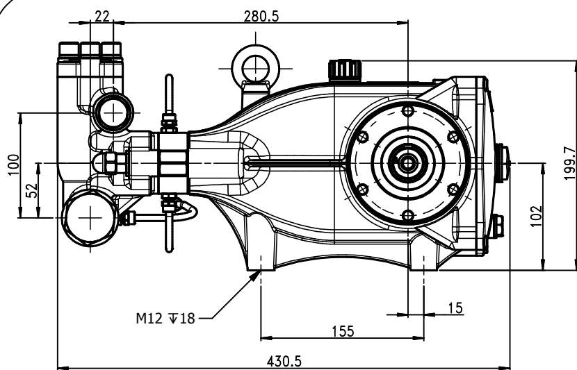
Dimensioni d'ingombro
